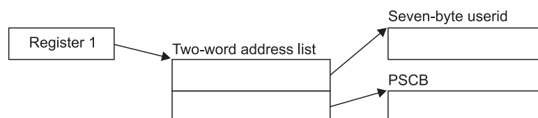
Figure 29. ERBT SOCK Input Parameter Structure
